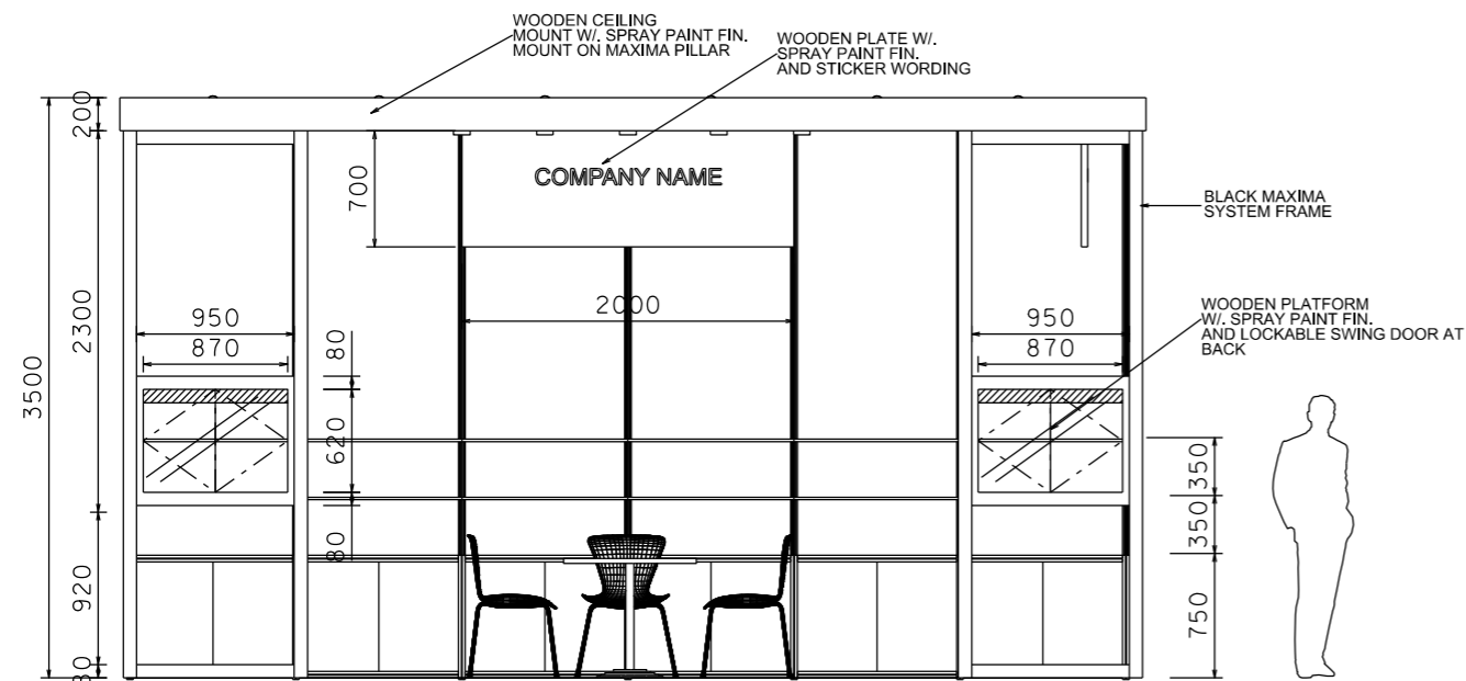
ELEVATION
