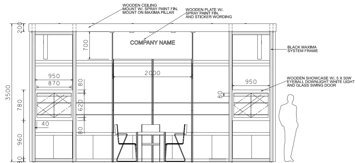
ELEVATION
