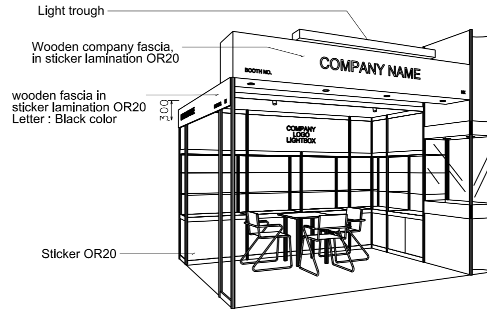
PERSPECTIVE N.T.S
